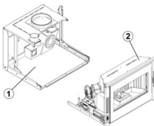
Fig. 25 - Structuur + machineromp
