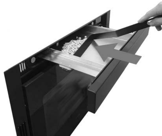
Fig. 35 - Duwen van de pellets met schep
