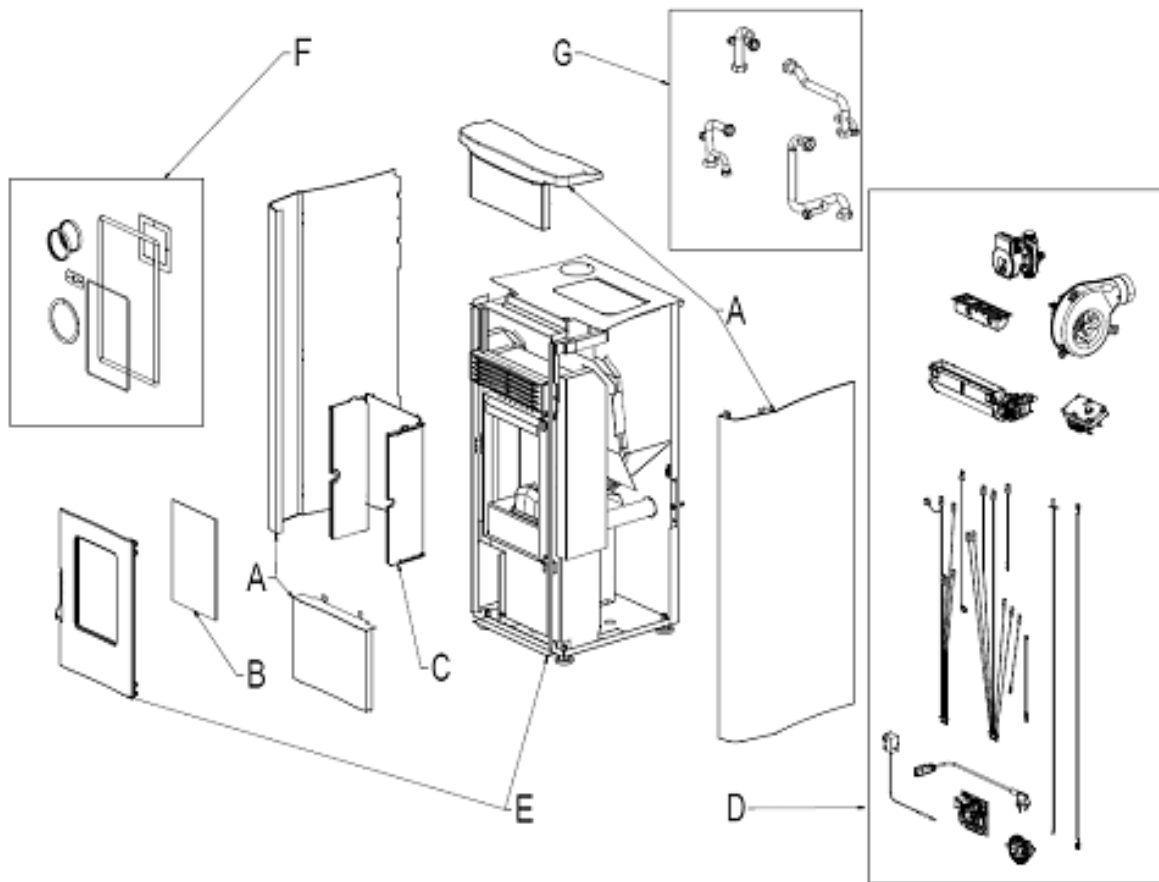
Fig. 1 - Dessin éclaté
