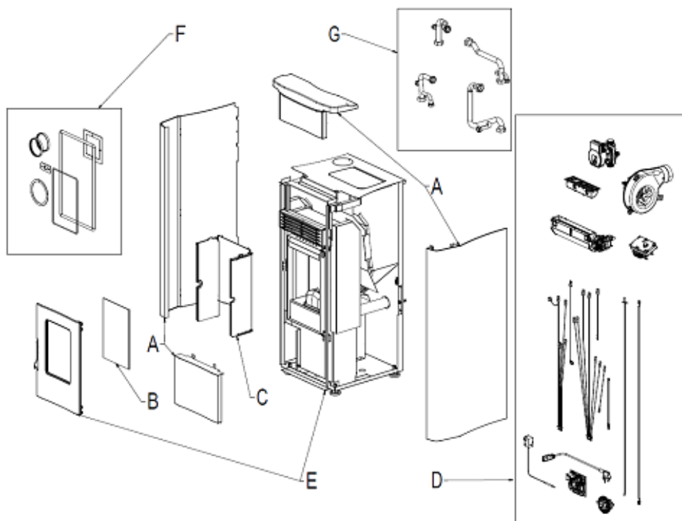
Fig. 1 - Esploso
