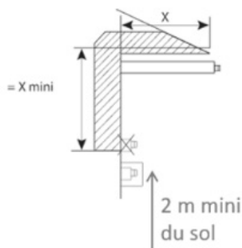
Fig. 14 - Rebord de toit
