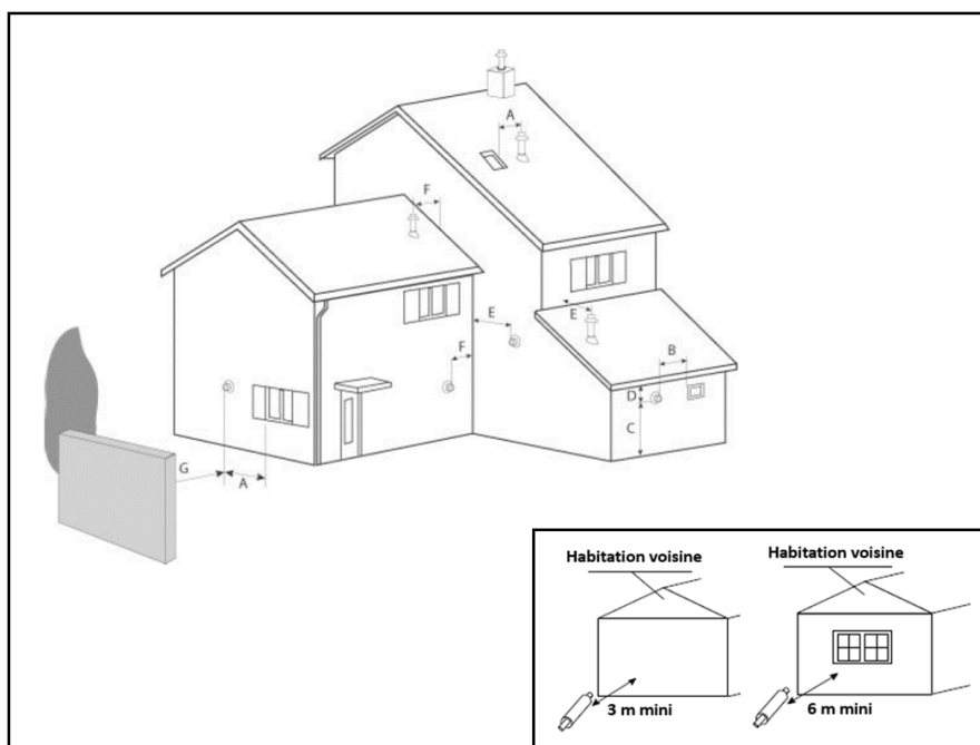
Fig. 13 - Position des terminaux
