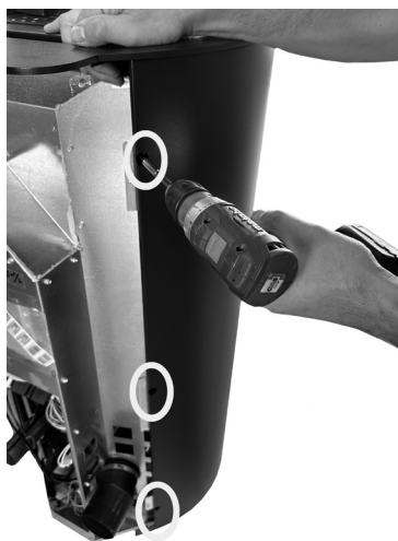
Fig. 28 - Retirer les vis.
