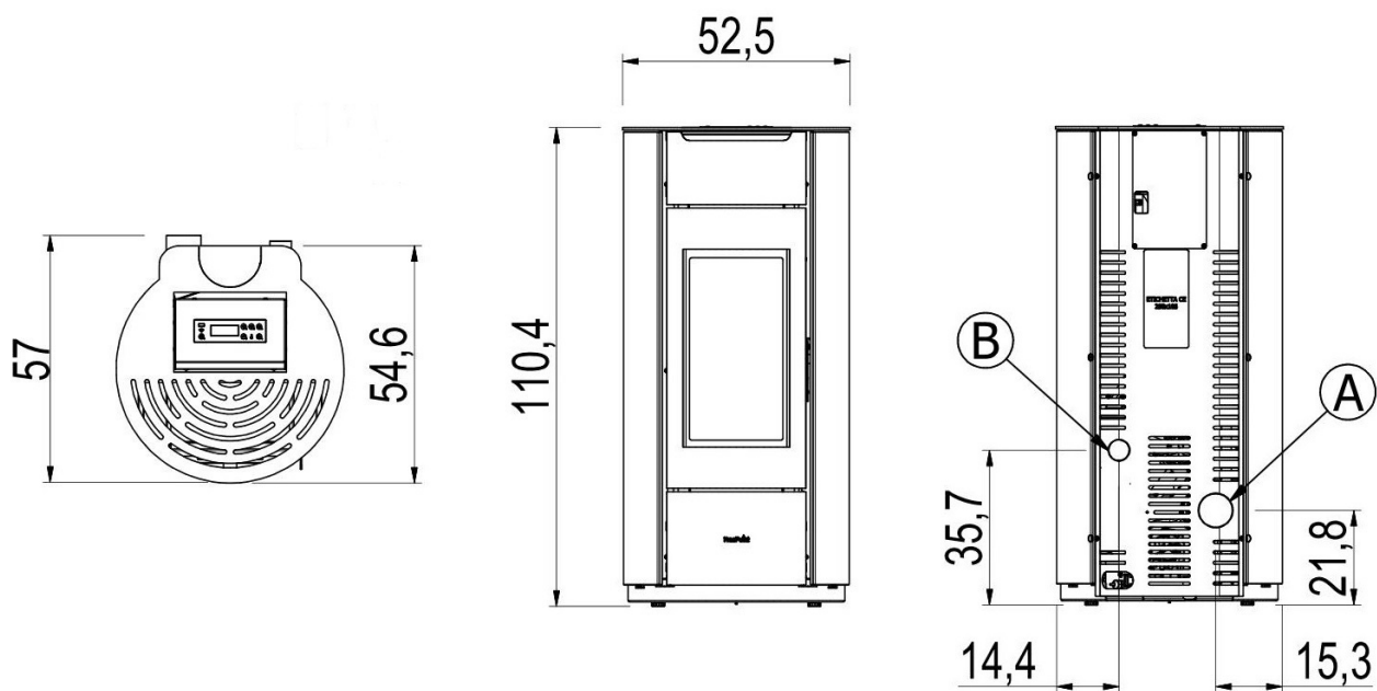
Fig. 22 - Dimensions générales: Eos 8 T1
