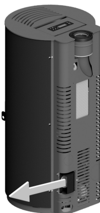
Fig. 39 - Spin
