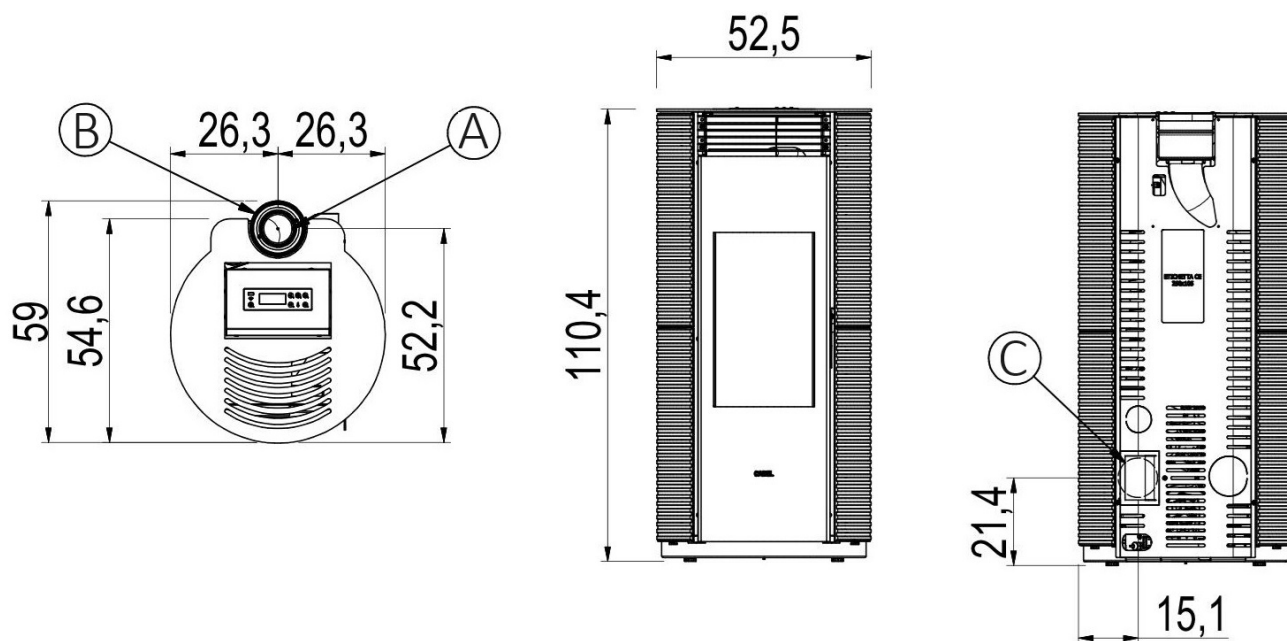
Fig. 21 - Dimensions générales: Spin Plus 9 Up-Twin T1
