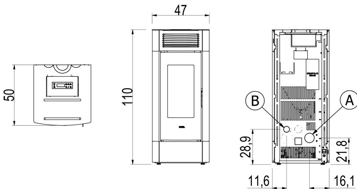
Fig. 23 - Cristal 9 Airtech T1
