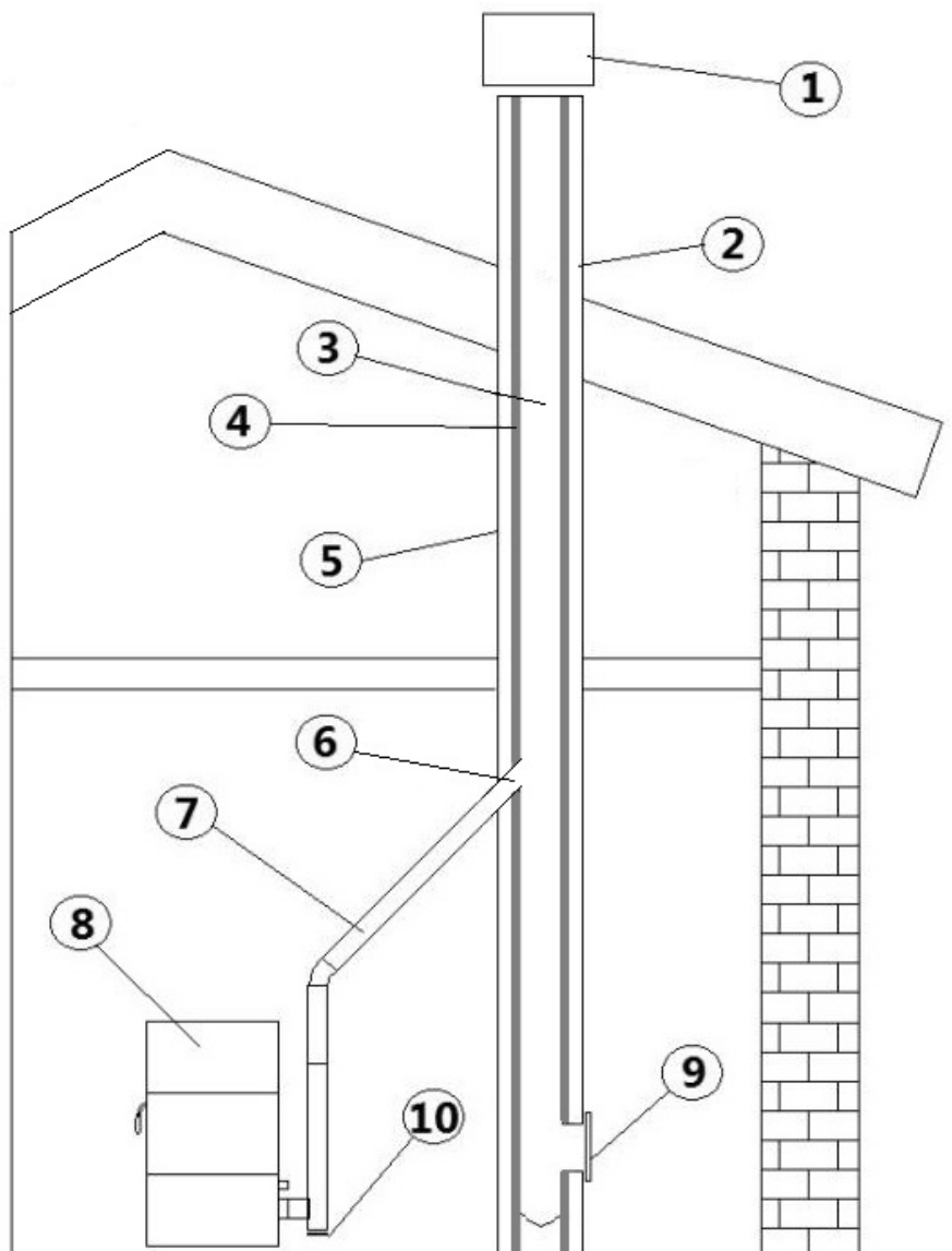
Fig. 2 - Composants de la cheminée
