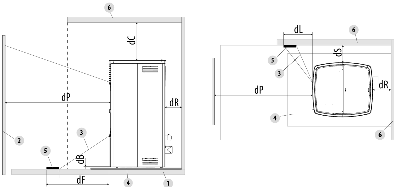
Fig. 20 - Distances de sécurité
